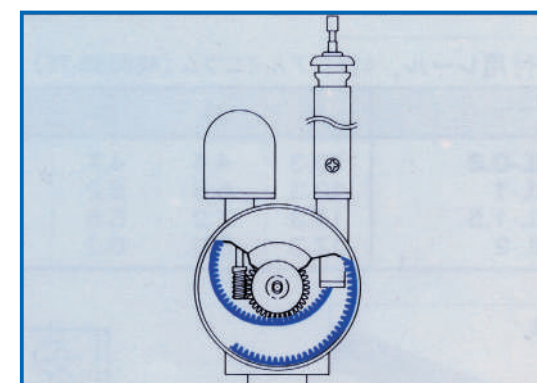
电动天线
